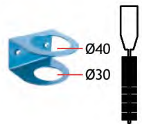
110 0 06 Blíster con 1 Unidad Para tenaza aberura múltiple
